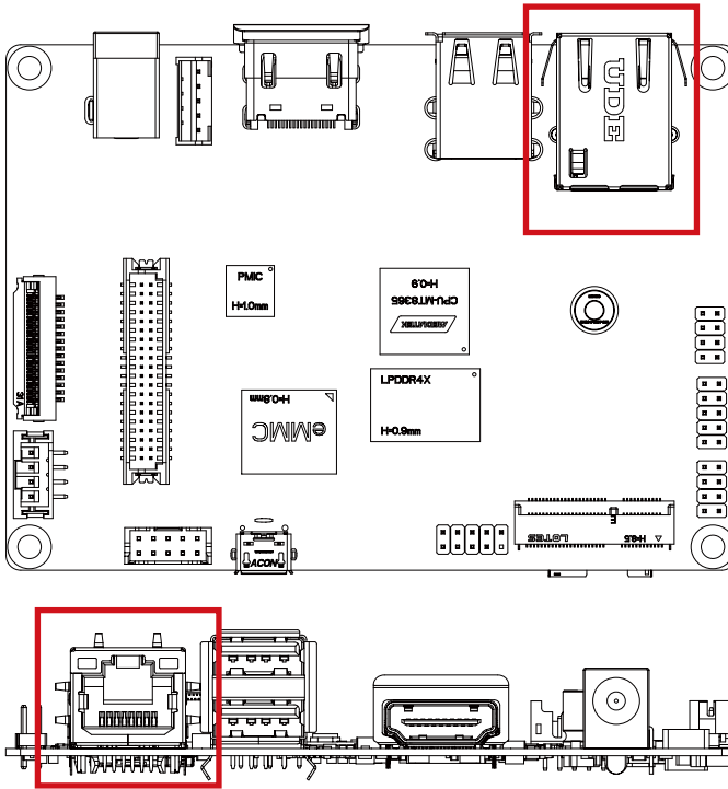
LAN Connector
