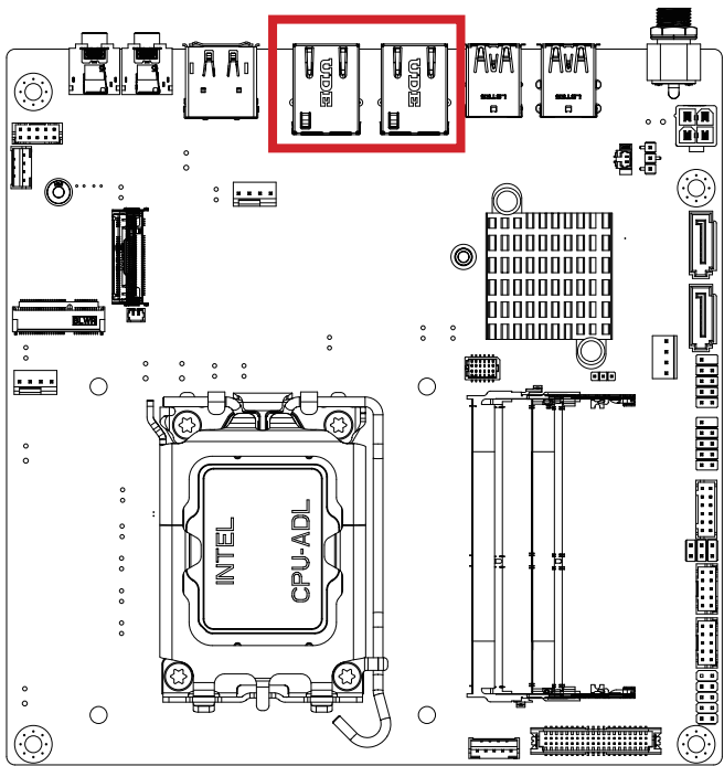
LAN Connector
